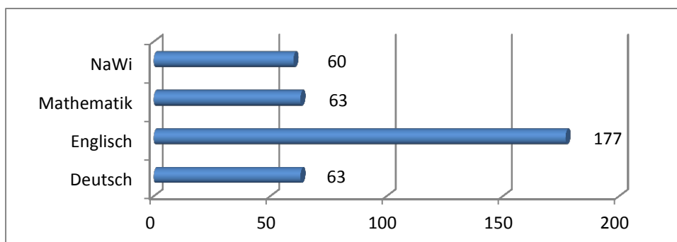
Grafik 2: Kompetenz- zuwachs in den getesteten Fächern von Klasse 5 nach Klasse 7
