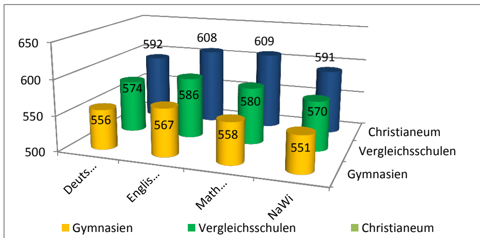
Grafik 1: KERMIT- Ergebnisse der 7. Klassen am Christianeum, den Vergleichs- schulen und allen Hamburger Gymnasien
